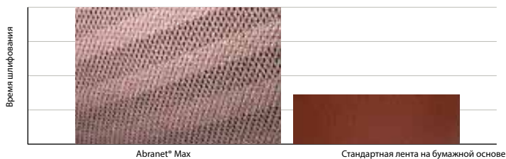
Сравнение Abranet® Max со стандартной лентой на бумажной основе P150
